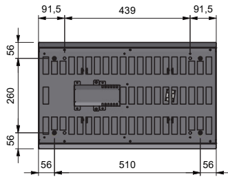
INFRA ER 3200
